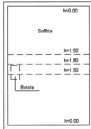
PIANO SECONDO (Sottotetto)
