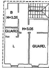
PIANO PRIMO
