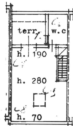
piano secondo (sottotetto)
