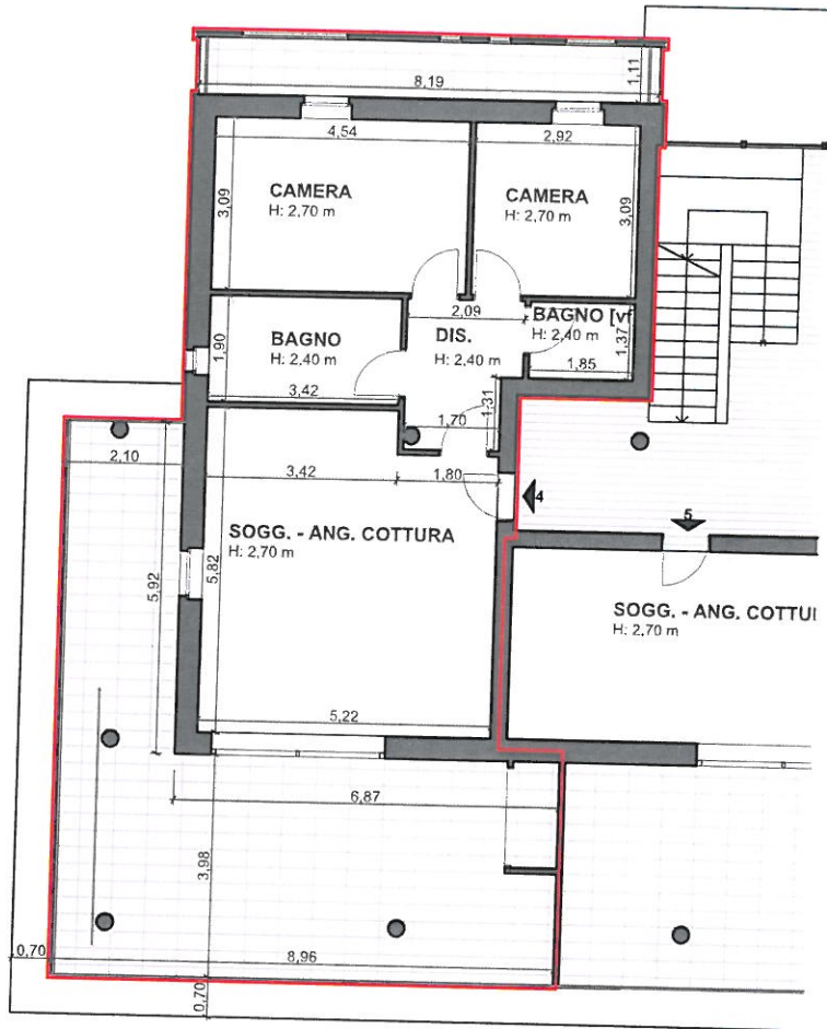
PIANTA PIANO PRIMO 1:100
